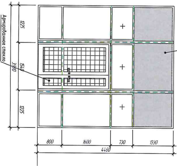
Заполнение сэндвич-панелями Выпукл. ВН-8
