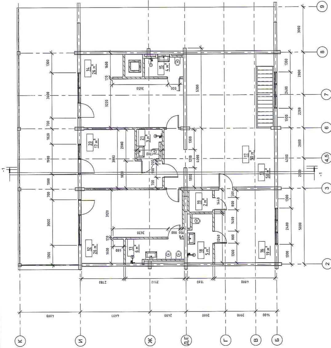
План второго этажа на о.м. 3,79
