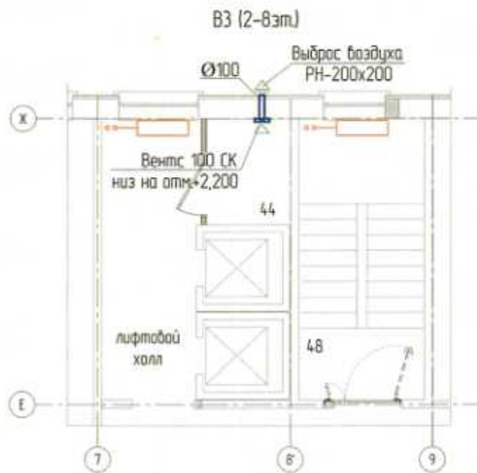
Фрагмент плана типового этажа (в осях Е-Ж и 7-9)
