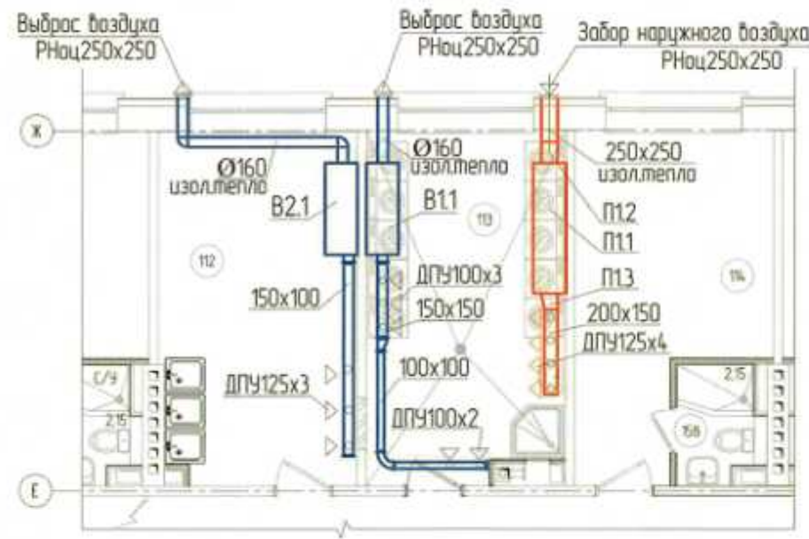
Фрагмент плана типового этажа (в осях Е-Ж и 7-9)
