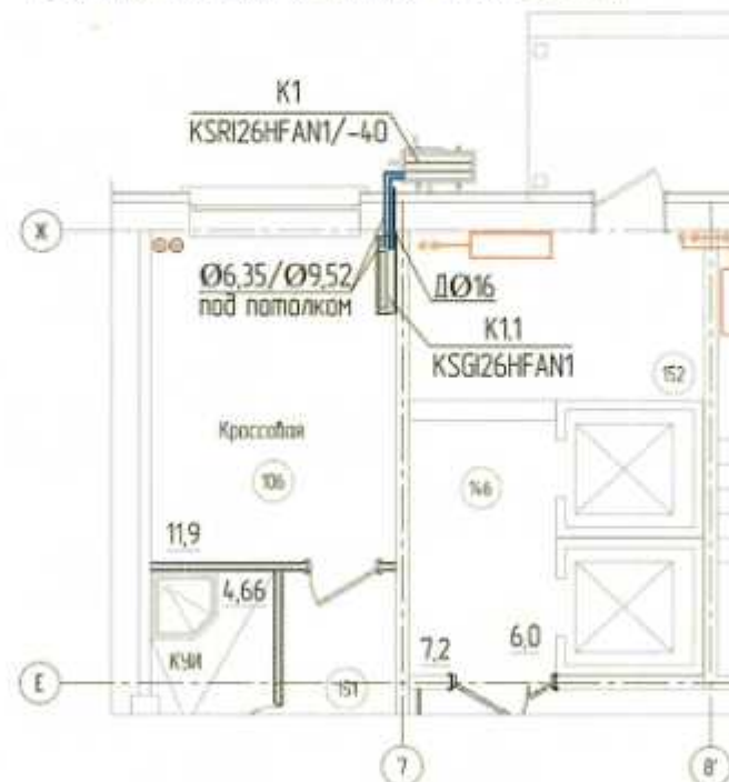
Кондиционирование. Фрагмент плана первого этажа (в осях Е-Ж и 7)
