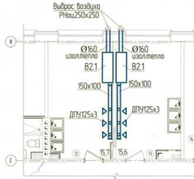
Фрагмент плана типового этажа (помещения кухни)
